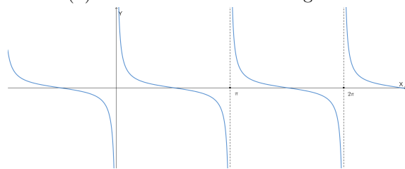
(d) Gráfica de la función cotangente
