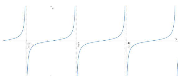
(b) Gráfica de la función tangente
