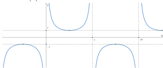
(c) Gráfica de la función cosecante
