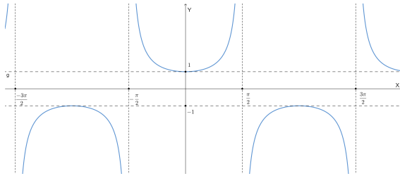
(a) Gráfica de la función secante
