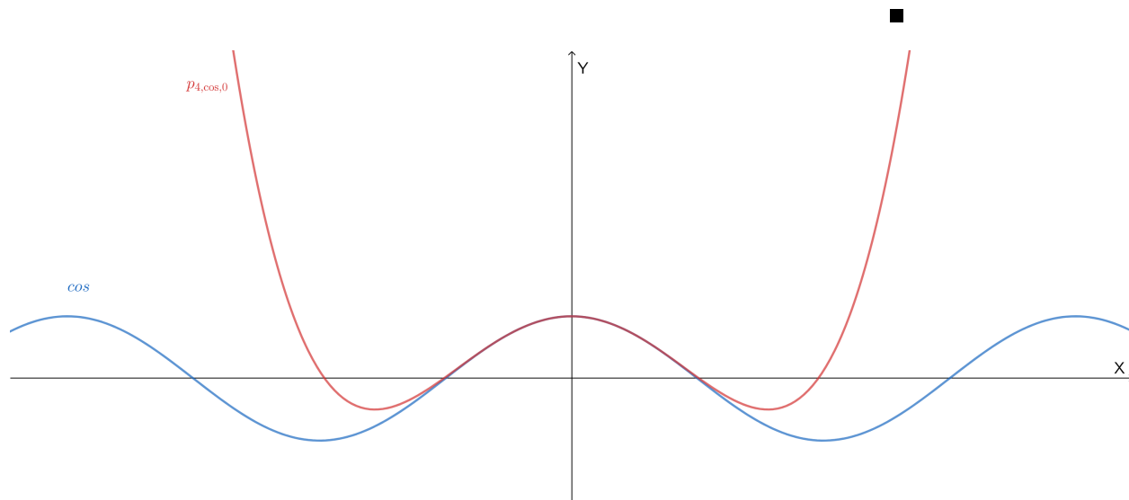
Figura 3: Se muestran las gráficas de \cos y de p_{4,\cos,0} .
