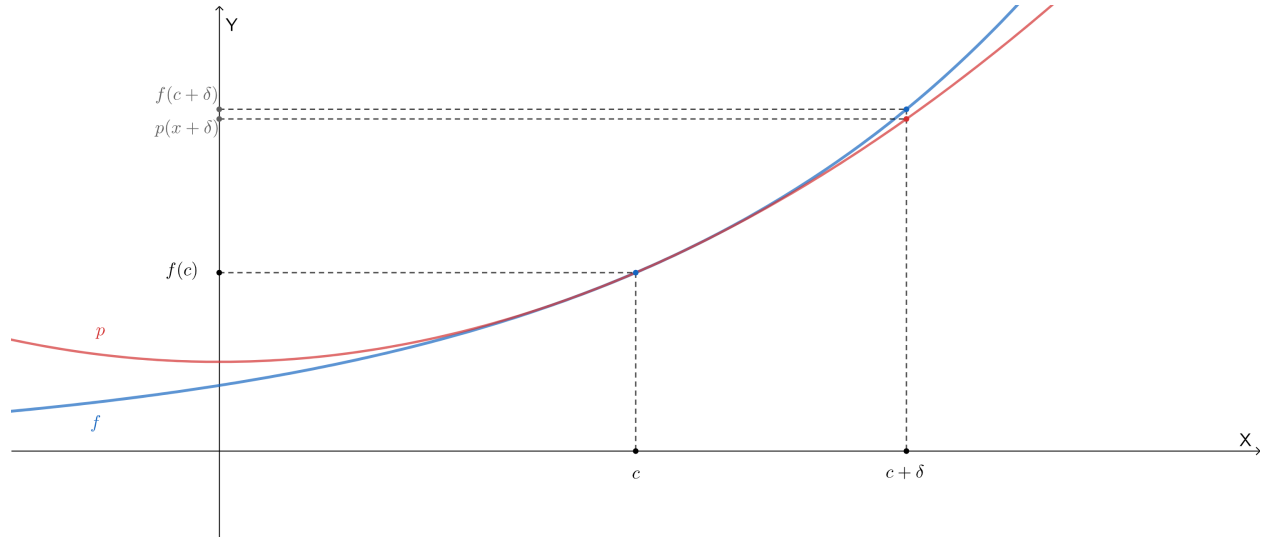
Figura 1: La función polinomial p se “aproxima” a la función f “cerca” de c y la diferencia entre f(c + \delta) y p(c + \delta) es muy “pequeña”
