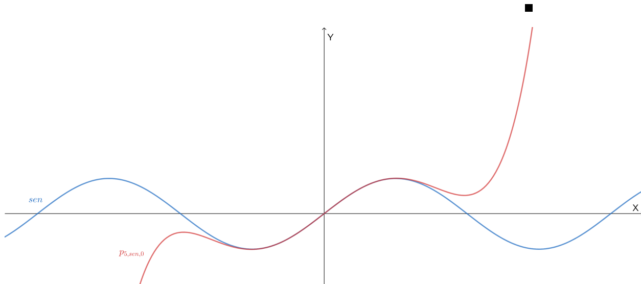
Figura 2: Se muestran las gráficas de \text{sen} y de p_{5,\text{sen},0} .
